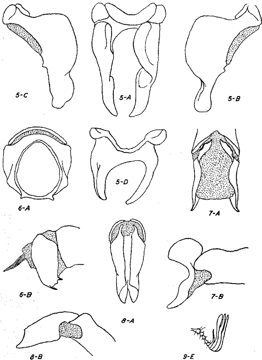
Fig. 5.— Phyllophaga chippewa , n. sp. Fig. 6.— Phyllophaga rossi , n. sp. Fig. 7.— Serica chicosnsis , n. sp. Fig. 8.— Serica sandiegensis , n. sp. Fig. 9.— Serica mendota , n. sp. A, En face view of male genitalia; B, lateral view of same; C, same; D, dorsal view of male genitalia; E, male antenna.
